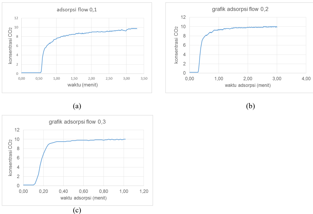
Gambar 1. Grafik adsorpsi CO 2 flow (a) 0,1 L/menit, (b) 0,2 L/menit, (c) 0,3 L/menit
