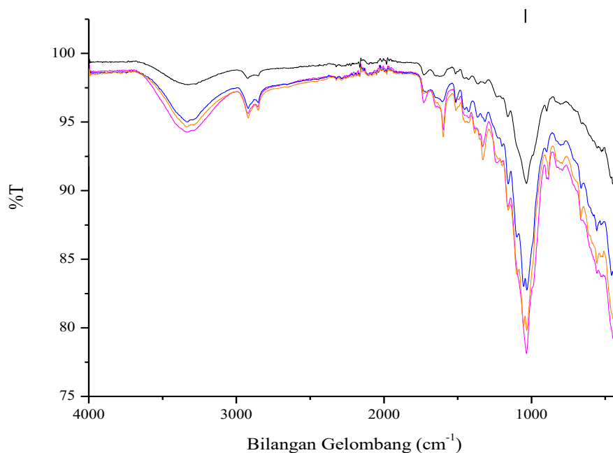
Gambar 6. Spektra FTIR Struktur Selulosa Aalang-alang
