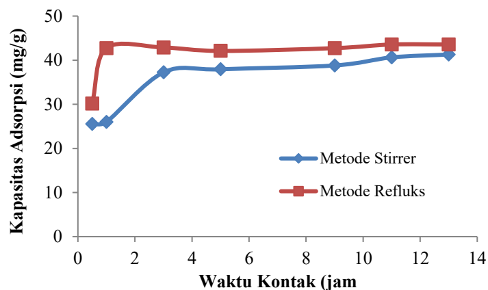
Gambar 4. Kurva Menunjukkan Waktu Kontak Optimum
