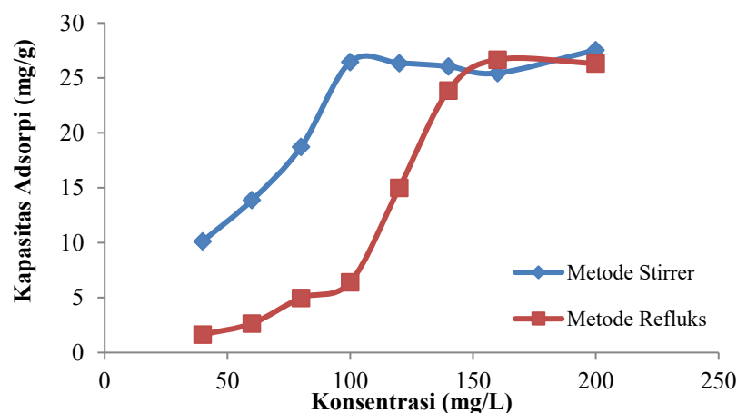
Gambar 5. Kurva Hubungan antara Kapasitas Adsorpsi dengan Konsentrasi
