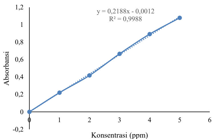
Gambar 2. Kurva Hubungan Absorbansi terhadap Konsentrasi
