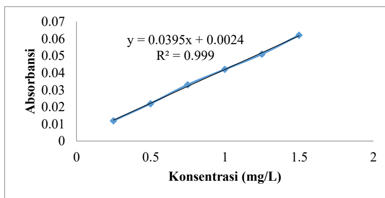
Gambar 1. Kurva Kalibrasi
